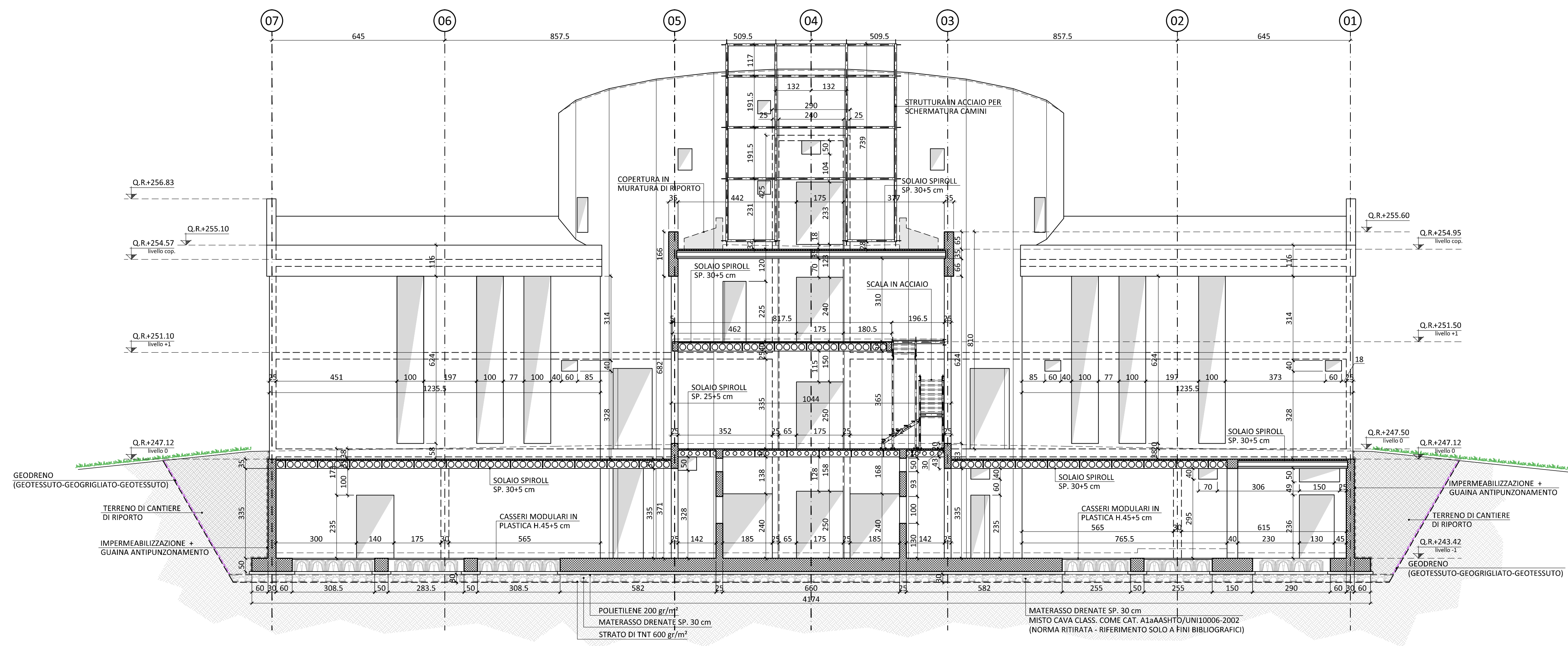
01 SEZIONE E-E SCALA 1:100
