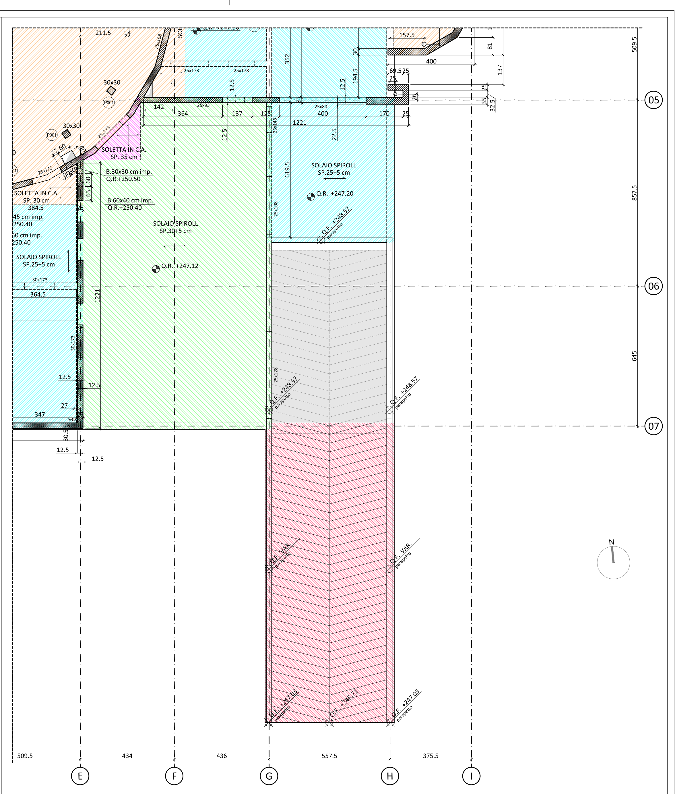
02 RAMP A SUD SCALA 1:100
